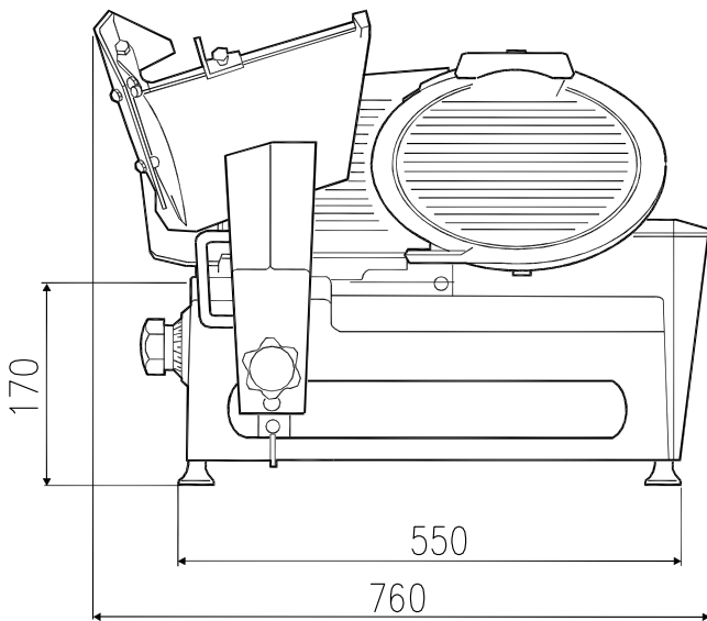
Oldalnézet
